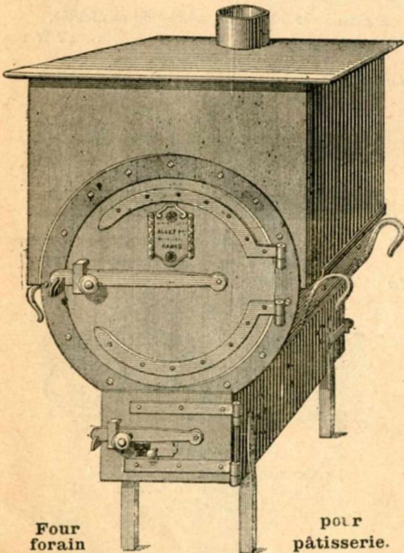
Four à pâtisserie carré, garni de briques réfractaires, foyer à bois.
