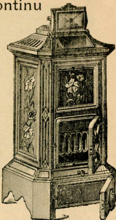
Calorifère anglais à feu visible, intérieur en terre réfractaire avec grille, porte au foyer, tuyau derrière. Nos 40 41 42 Hauteur..... 0.97 1.08 1.21 Fonte noire..... 80 fr. 95 fr. 112 fr. Fonte émaillée noire. 105 fr. 135 fr. 165 fr.
