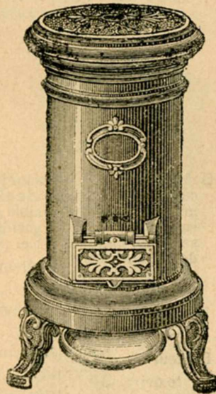
Calorifère rond tout fonte, tuyau derrière avec barette, intérieur terre réfractaire sans grille.
