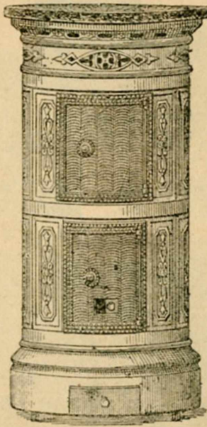
Calorifère rond à socle avec tablette en marbre et four, portes en fonte, bois et charbon. Diamètre du corps.. 0.30 0.33 0.36 0.39 0.42 Hauteur..... 0.80 0.86 0.89 0.93 0.98 Faïence blanche à four. 62f. 68f. 76f. 85f. 96f. — couleurs à four.. 77f. 86f. 96f. 108f. 123f. — blanche à bouches. 65f. 72f. 80f. 89f. 99f. — couleurs à bouches. 72f. 82f. 92f. 102f. 115f.
